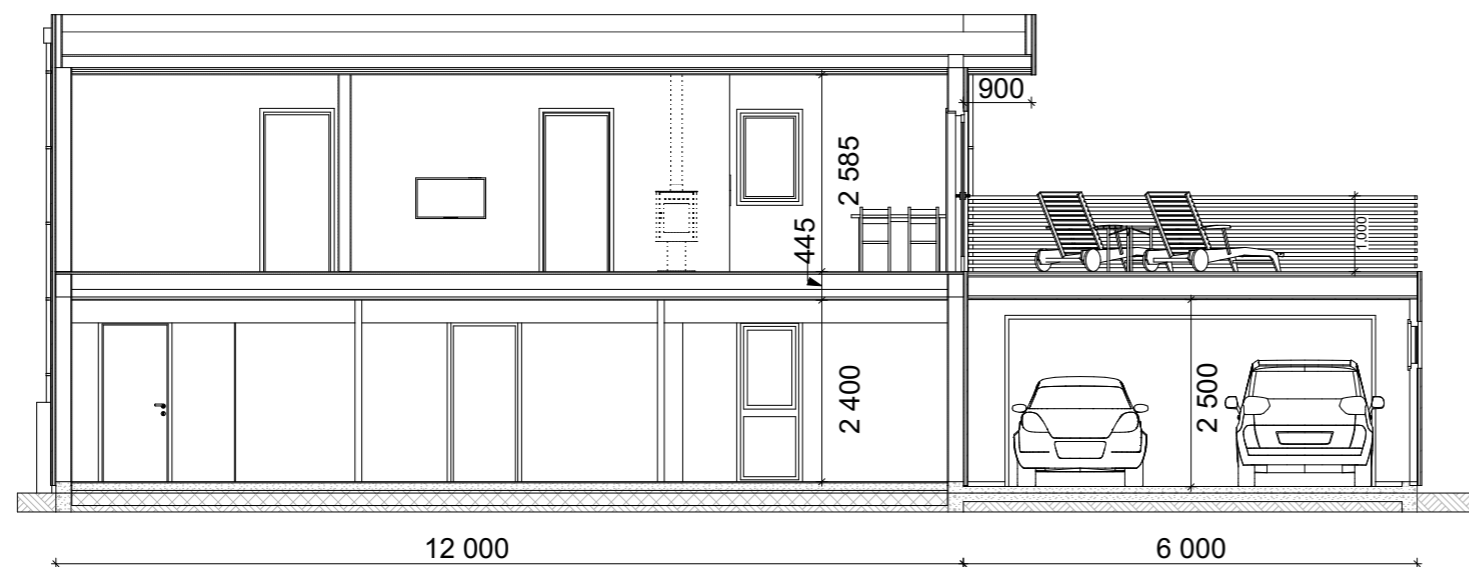
Snitt B-B
