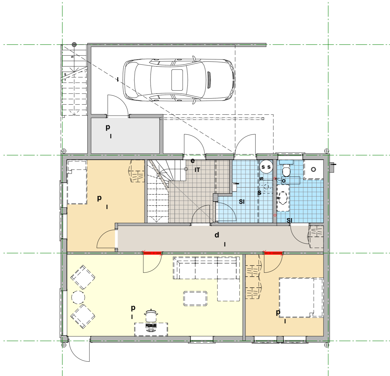
Innredet 1. etasje, rettvendt
