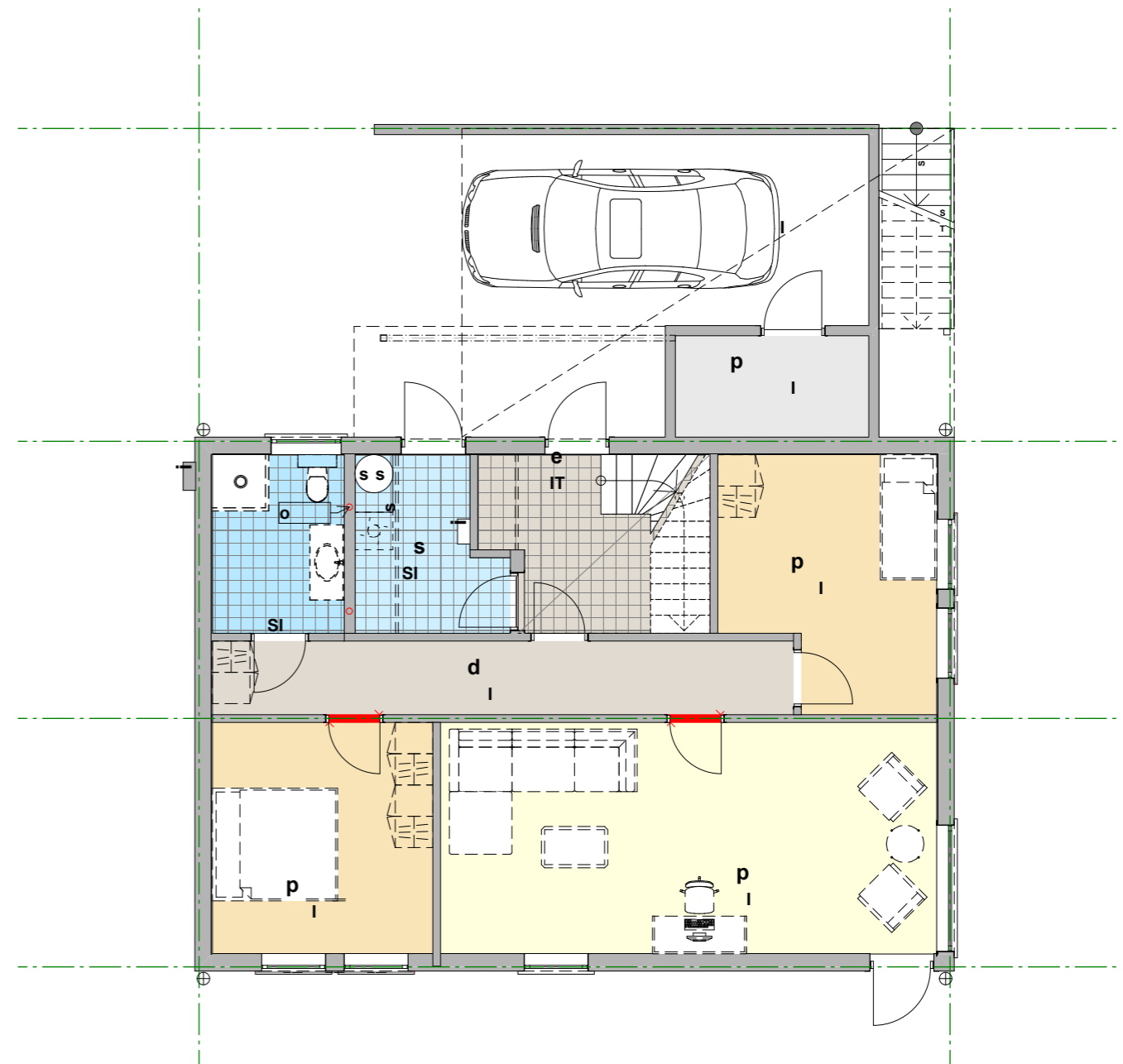
Innredet 1. etasje, speilvendt
